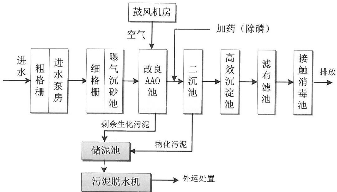
图2.2-1 阳春市岗美镇生活污水处理厂处理工艺流程图
