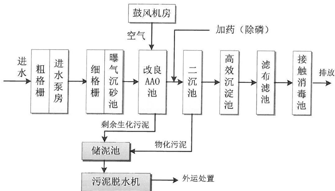
图2.2-1 阳春市合水镇生活污水处理厂处理工艺流程图
