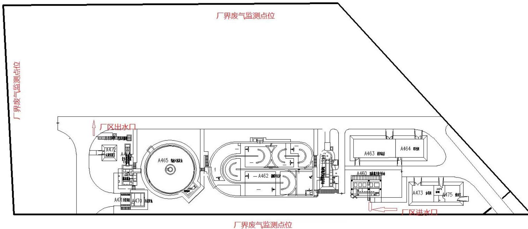
附图 6 项目总平面布置图
