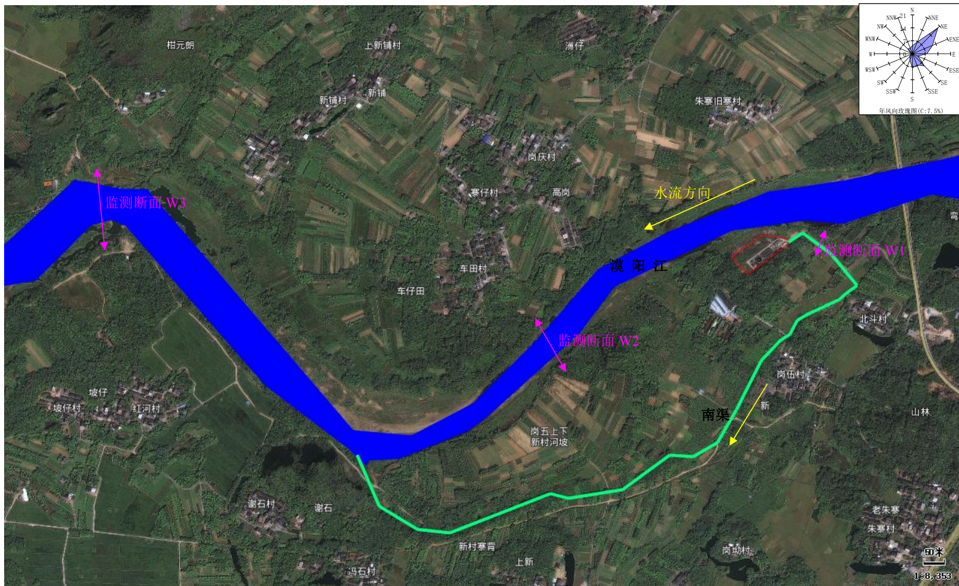
附图 8 水质现状监测布点图
